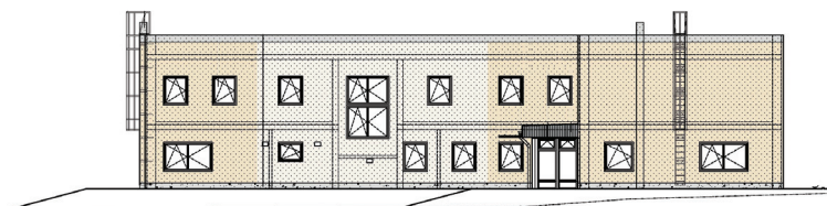
POHLED OD VÝCHODU M 1 : 100
