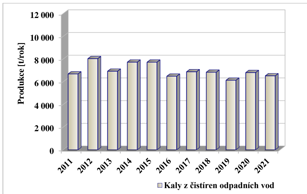
Graf č. 26: Celková produkce kalů z čistíren odpadních vod v letech 2011 – 2021.
