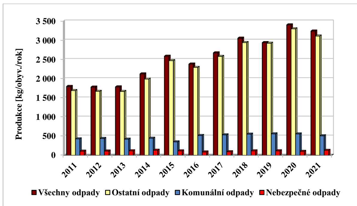
Graf č. 3: Produkce odpadů na obyvatele v letech 2011 – 2021.
