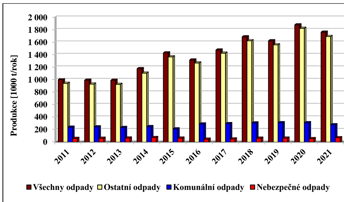
Graf č. 1: Celkové produkce odpadů v letech 2011 – 2021.
